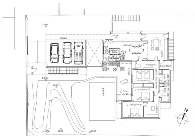
ANTEPROYECTO DE VIVIENDA UNIFAMILIAR NIVEL 1
